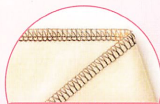
4本糸合わせ縁かがり縫い
